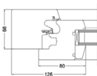
DETTAGLIO LATERALE FINESTRA CON PROFILATURA ANTA STANDARD
