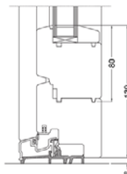
DETTAGGIO INFERIORE PORTAFINESTRA CON PROFILATURA ANTA STANDARD
